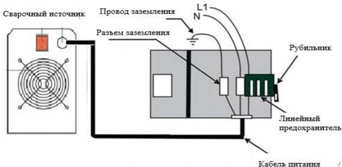
Рисунок 1 Применение предохранителя.
